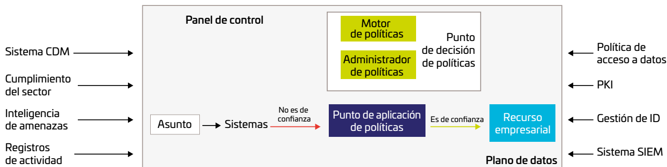
Figura 1: Enfoque de la arquitectura Zero Trust centrada en la identidad del NIST. Fuente: NIST SP 800-207
